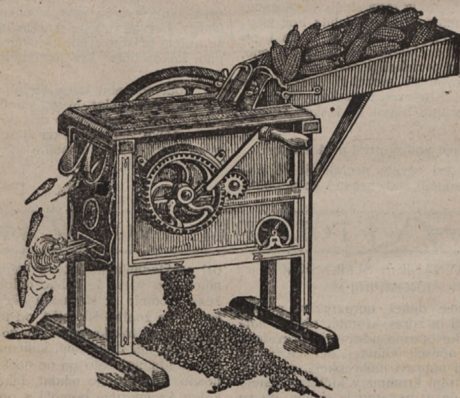
Sliki predstavljata dva tipa robkalnika za koruzo.
