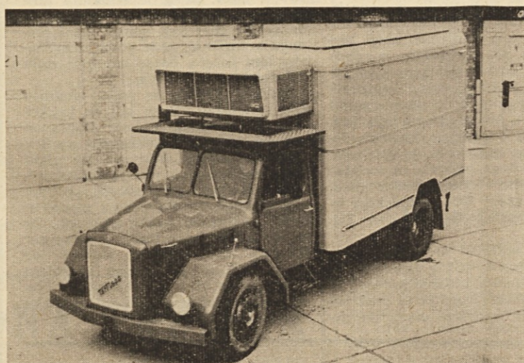
Kamion-hladilnik „TAM 4500 HS“ z agregatom
