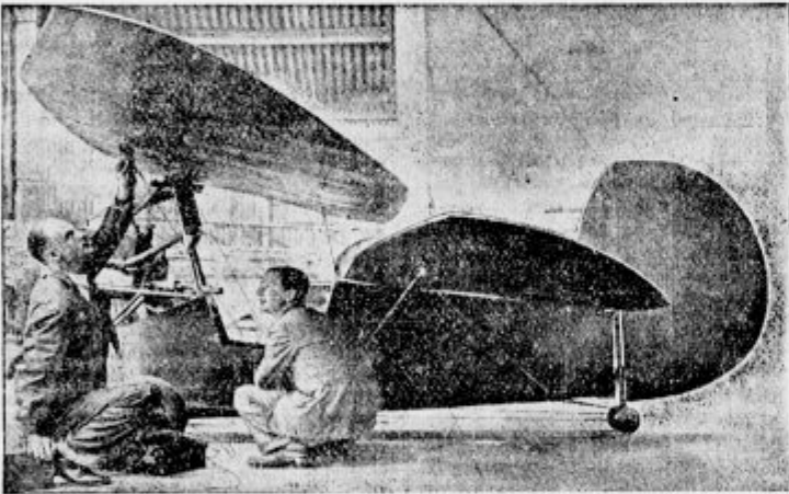
Kolo-letalo. Neki 23 letni Anglež je izumil to letalo, ki bo pač najmanjše in najcenejše letalo sveta. Dolgo je 360 cm, široko 480 cm, ima 12 konjskih sil, napravi 108 km na uro in stane približno 19.000 dinarjev.
