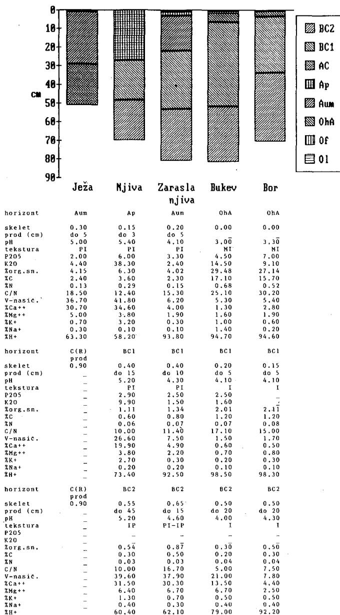
Slika 9: Primerjava fizikalno-kemijskih lastnosti petih značilnih talnih profilov v Mučki Dobravi
