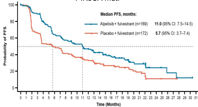
PIK3CA mut.
