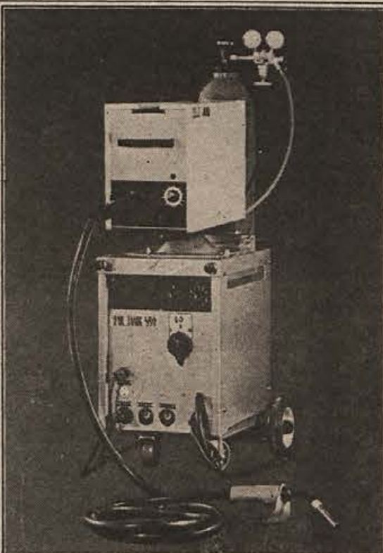
A 10-275 uređaj za poluavtomatsko zavarivanje A 10-275 i A 10-400
