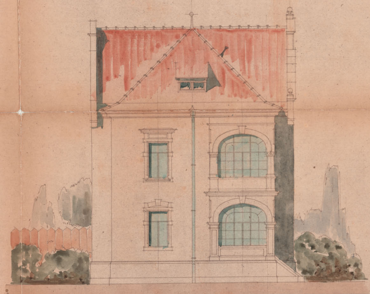
WESTL. ANSICHT
