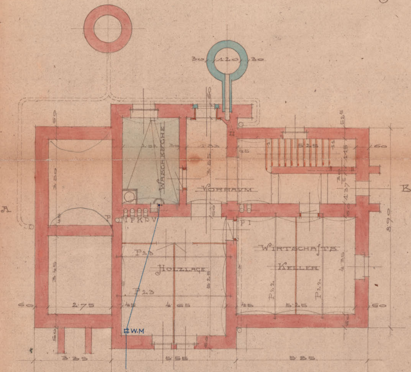
KELLER
