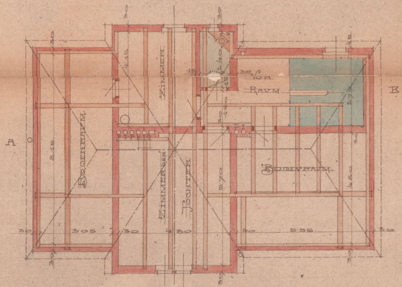
DACHBODEN
