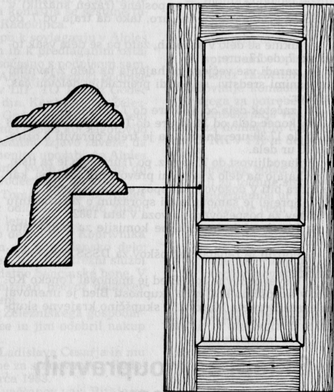
Stilna vrata S-3 Krilo z izrezom z ukrivljeno zgornjo letvijo
