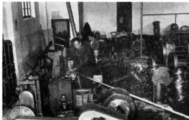
Na fotografiji: Proizvodnja gibljivih cevi v Klemosovem obratu v Voličini. Foto: M. Brumen
