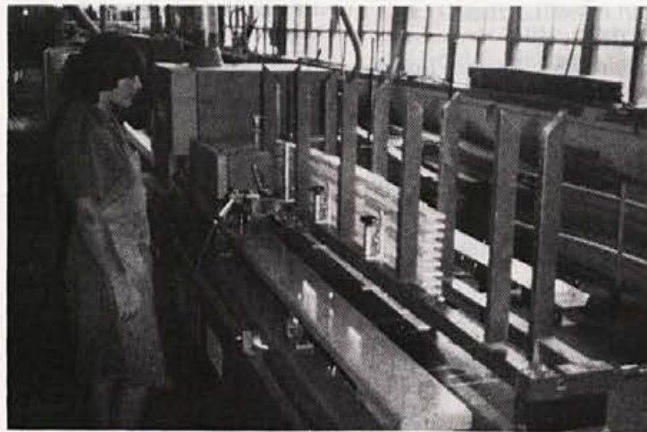
Avtomatska izdelava sredic za tekaške smuči
