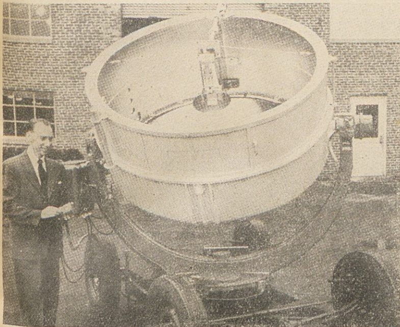
Sončna peč. Uporabljajo jo v raziskovalne namene za izpostavljanje materialov temperaturam do 3.500 °C. Napravo z izkoriščanjem sončne energije bodo v prihodnosti uporabljali za ogrevanje domov in pri raznih kemičnih reakcijah
