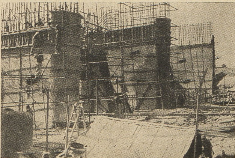
Gradišče hidrocentrale Gujranwala v pokrajini Lahore v Pakistanu
