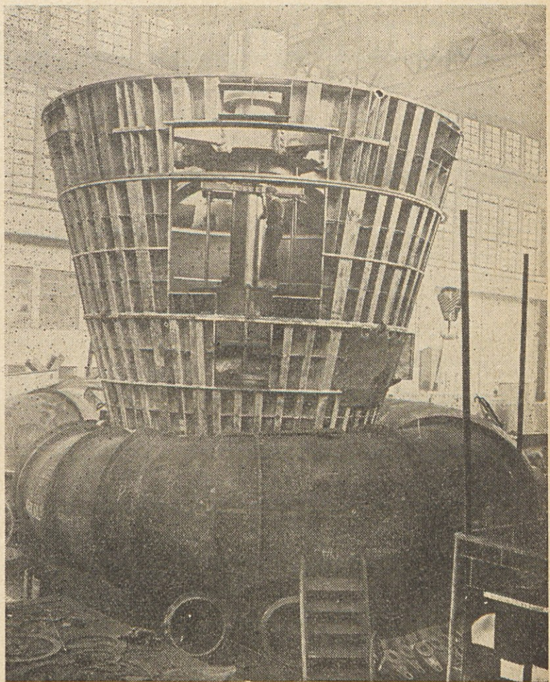
Delavniška montaža Francisove turbine za HE Peručo
