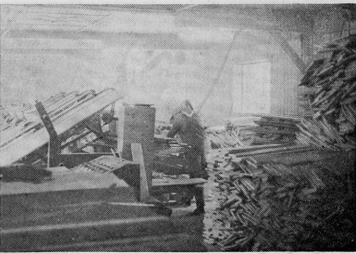
Delo na formatni krožni žagi
