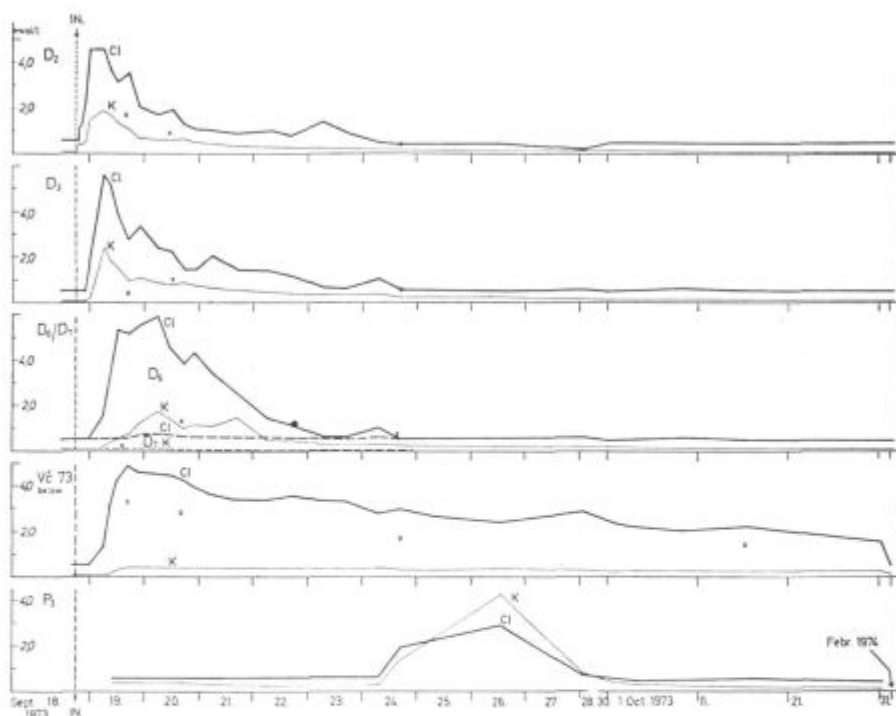
Krivulje koncentracije za kalij in klor v piezometrih D 2, D 3, D 6, D 7, Vč 73 in P 1. Krivulja za klor — debelo, za kalij tanko izvlečena; vrednosti v piezometru D 7 črtkasto; križci = zvišanje totalne trdote v mval/l v primerjavi z začetno vrednostjo; IN — čas injiciranja kalijeve soli.
