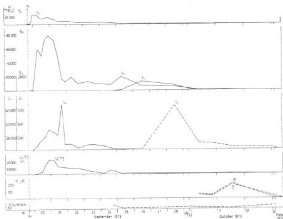
Krivulje koncentracije za uranin v piezometrih S_2 , S_3 , S_5 , S_6 , S_7 , Vč/73 , P_3 in P_4 in v studencu. IN — čas injiciranja za uranin. Opozarjamo na različno časovno skalo za 19.—28. september in 29. september do 31. oktober 1973.
