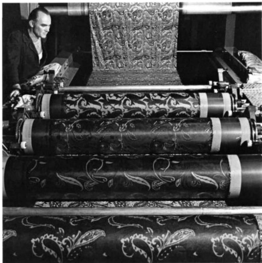
Tekstilna tovarna Prebold — nov tiskarski stroj z vrtljivimi šablonami
