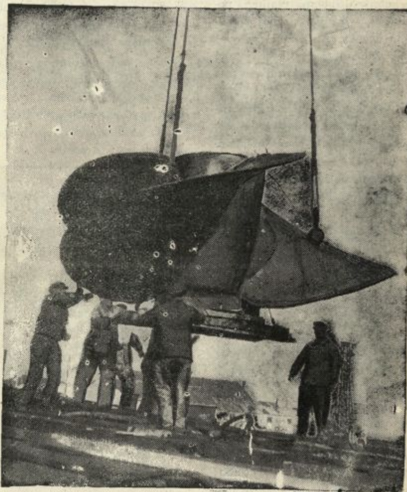
Za novi francoski prekomornik »NORMANDIE«, ki bo oskrboval promet na progi Le Havre - New York. Vijak tehta 23 ton.
