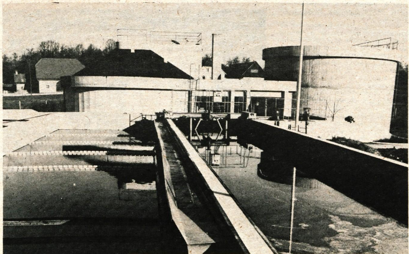
Centralna čistilna naprava (odprli so jo aprila lani) predstavlja prvi resnejši korak k zaščiti voda in nasploh okolja v Škofji Loki. Vanjo je speljanih že večina odtočnih kanalov iz posameznih četrti mesta. Letos bodo podoben, le nekoliko manjši objekt začeli graditi tudi v Železnikih. – Foto: F. Perdan
