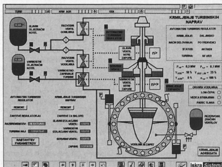
Operaterjev nadzor nad delovanjem agregata
