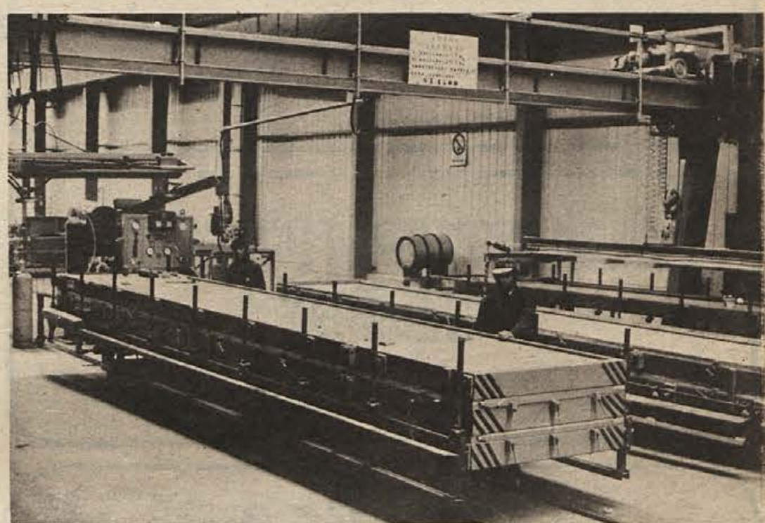
Naprava za izdelovanje fasadnih plošč
