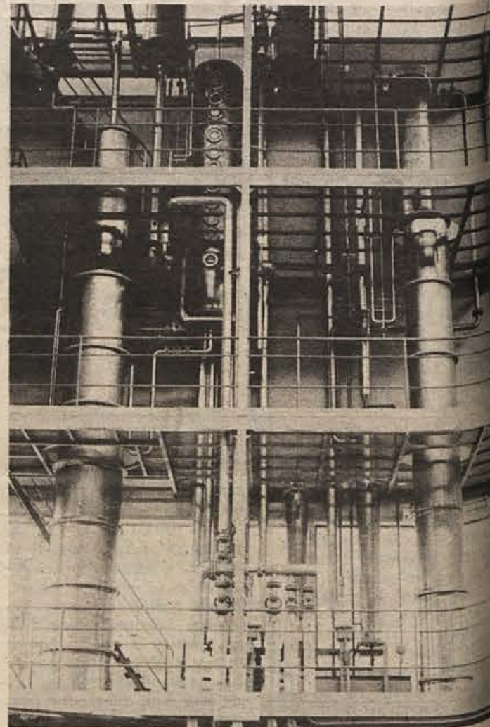
Del destilacijskih naprav (Foto: M. Vesel)
