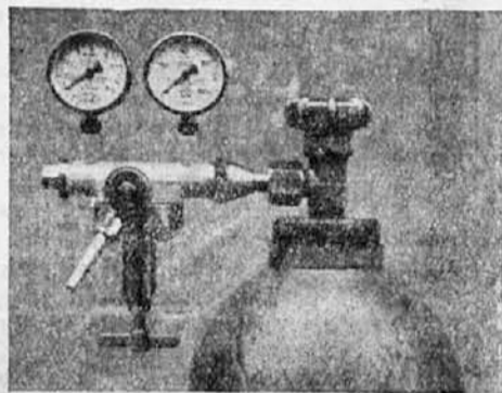
REDUČNI VENTIL »AGA-RUŠE« Z NAVZDOL OBRNJENIM REGULIRNIM VIJAKOM.
