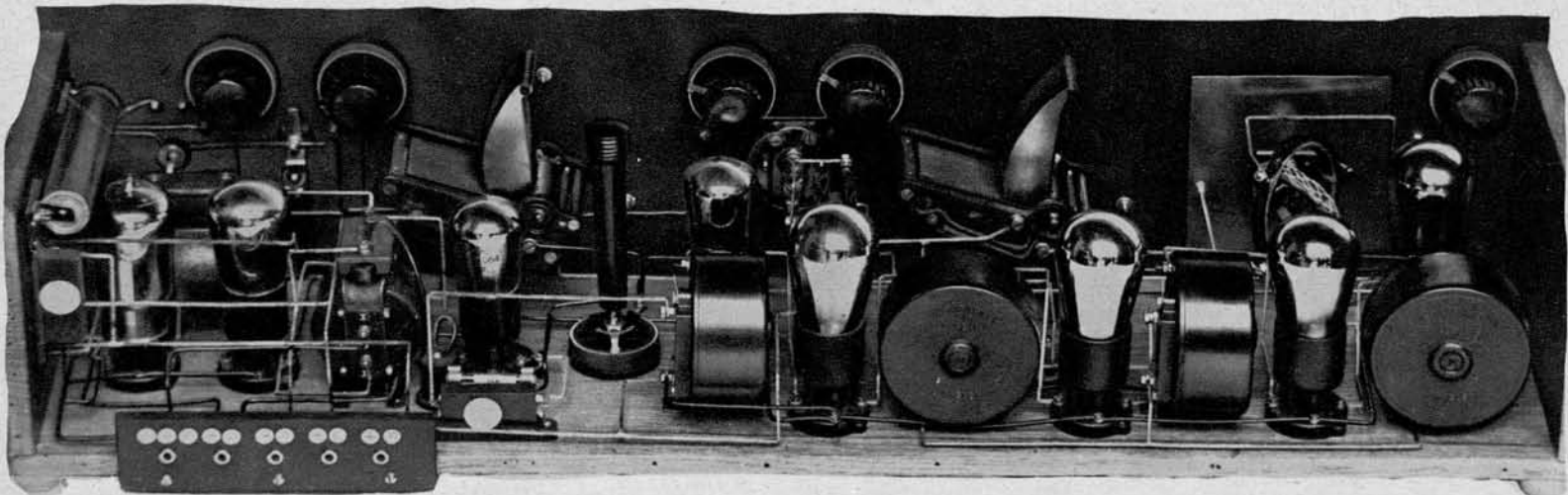
Osemcevni sprejemni aparat za okvirno anteno.
