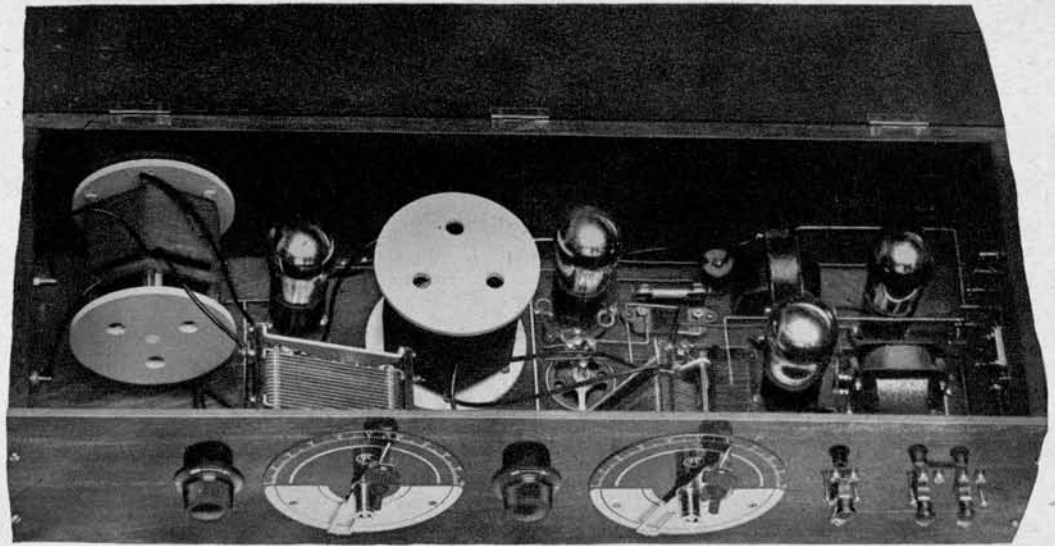
Štiricevni radijski sprejemni aparat za visoko anteno.
