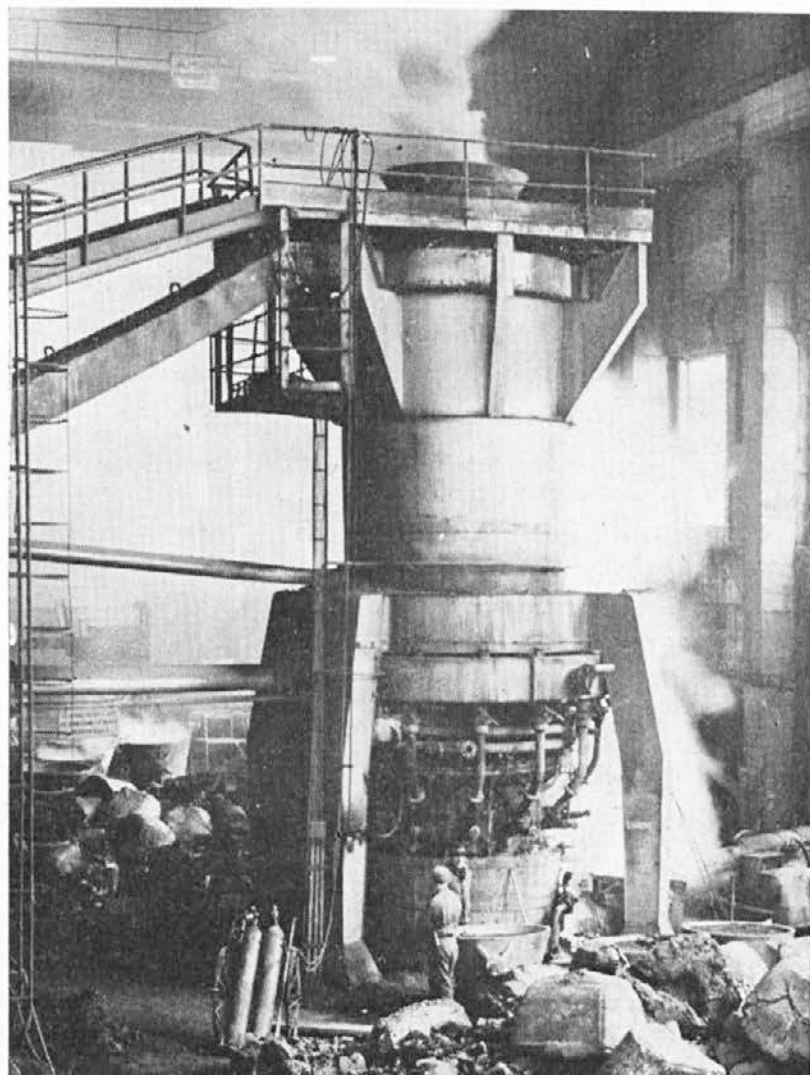
Visoka peč
