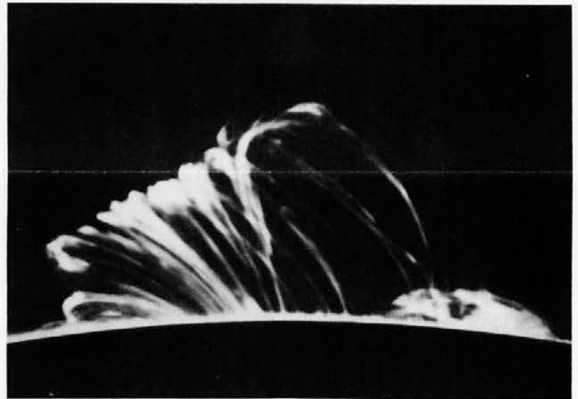
Magnetne arkade, ki so posledica sončnega blišča na sončnem robu. Fotografija je iz poljskega astronomskega observatorija v Wroclavu
