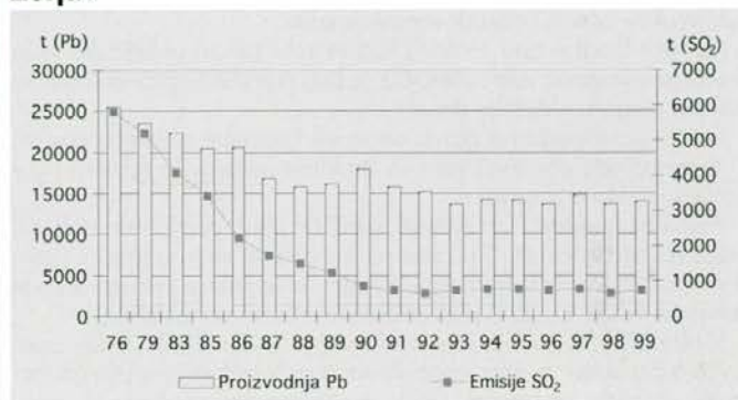
Graf 1 : Proizvodnja svinca in emisije SO 2 v topilnici Žerjav
