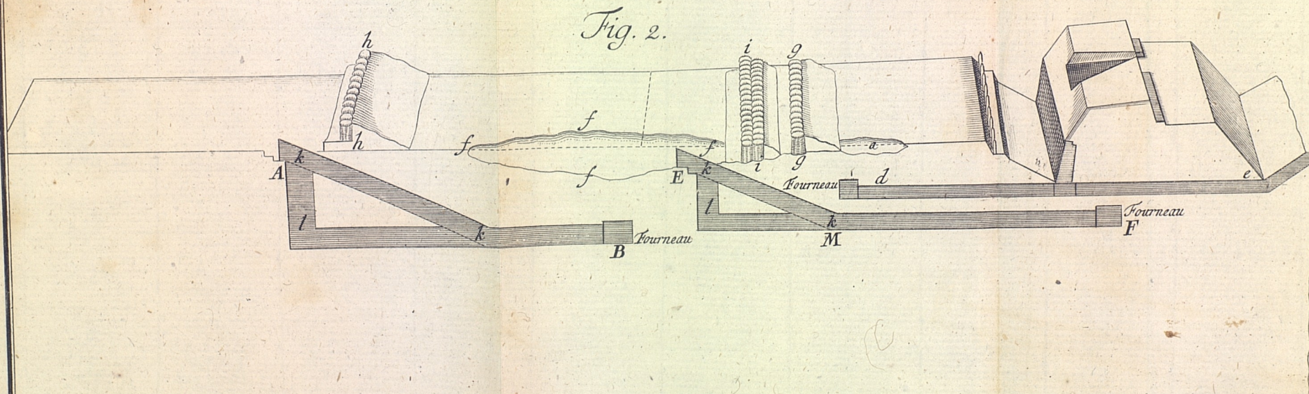
Profil der Sappen, Minen und der Entonnoirs wie auch des Forts N o 2.
