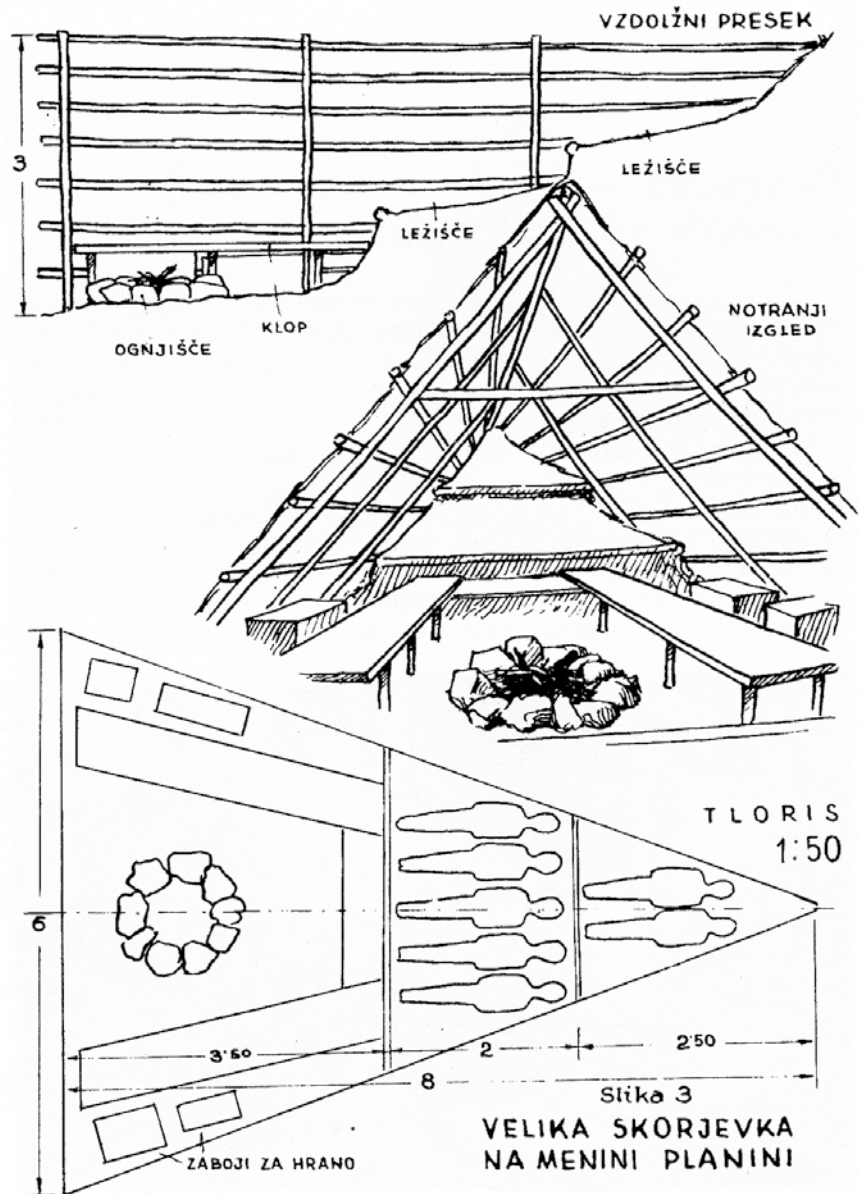
Notranja ureditev škorjevke. Gradivo iz knjige Miloša Mehore »Drvarske kočé na Slovenskem« iz leta 1946.
