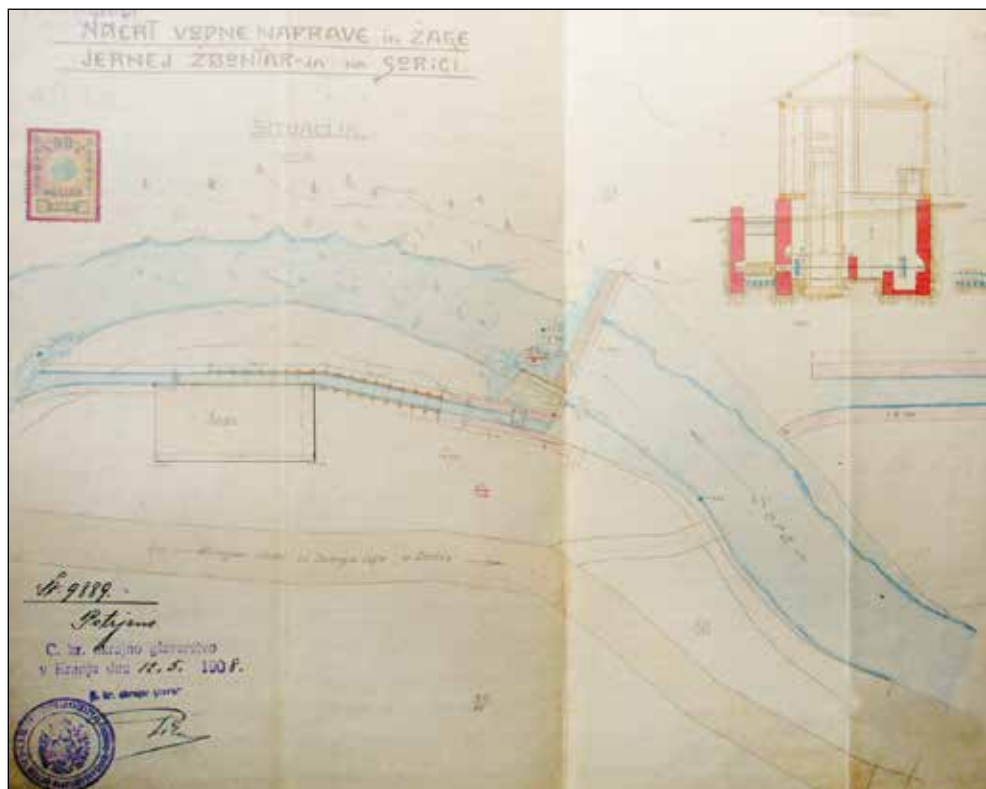
Pogled na situacijo terena s severne strani, profili ter tloris žage po načrtu leta 1908.
