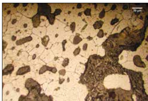
Slika 24. Metalografska analiza kovnega železa iz volka, pridobljenega pri taljenju 2017 v Železnikih. Leva slika nakazuje področje, kjer je prevladujoča feritna struktura s številnimi vključki žlindre. Desna slika nakazuje področja s prevladujočo perlitno strukturo, na meji z žlindro pa je prišlo do razogličenja in se nahaja ferit. Foto: Barbara Bertoncelej
