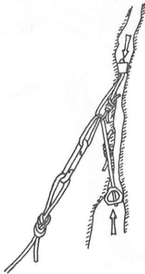
Kombinacija dveh zatičev v navpičnih počeh
