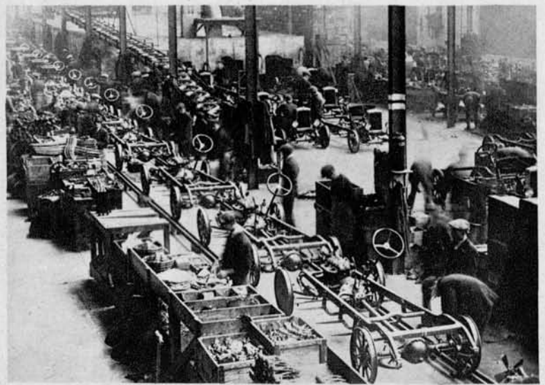
Pogled v tvornice avtomobilov Cowley , kjer izdelajo po Taylorjevem sistemu na tekočem traku 200 avtomobilov dnevno.
