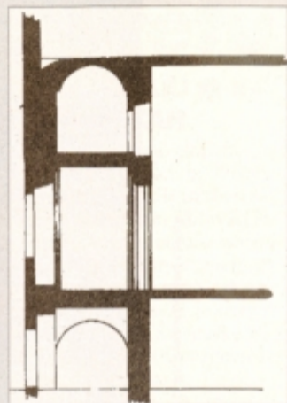
Prezrez skozi vzhodni del cerkvene ladje, pogled s severne strani; risal: B. Vnuk, M 1: 100
