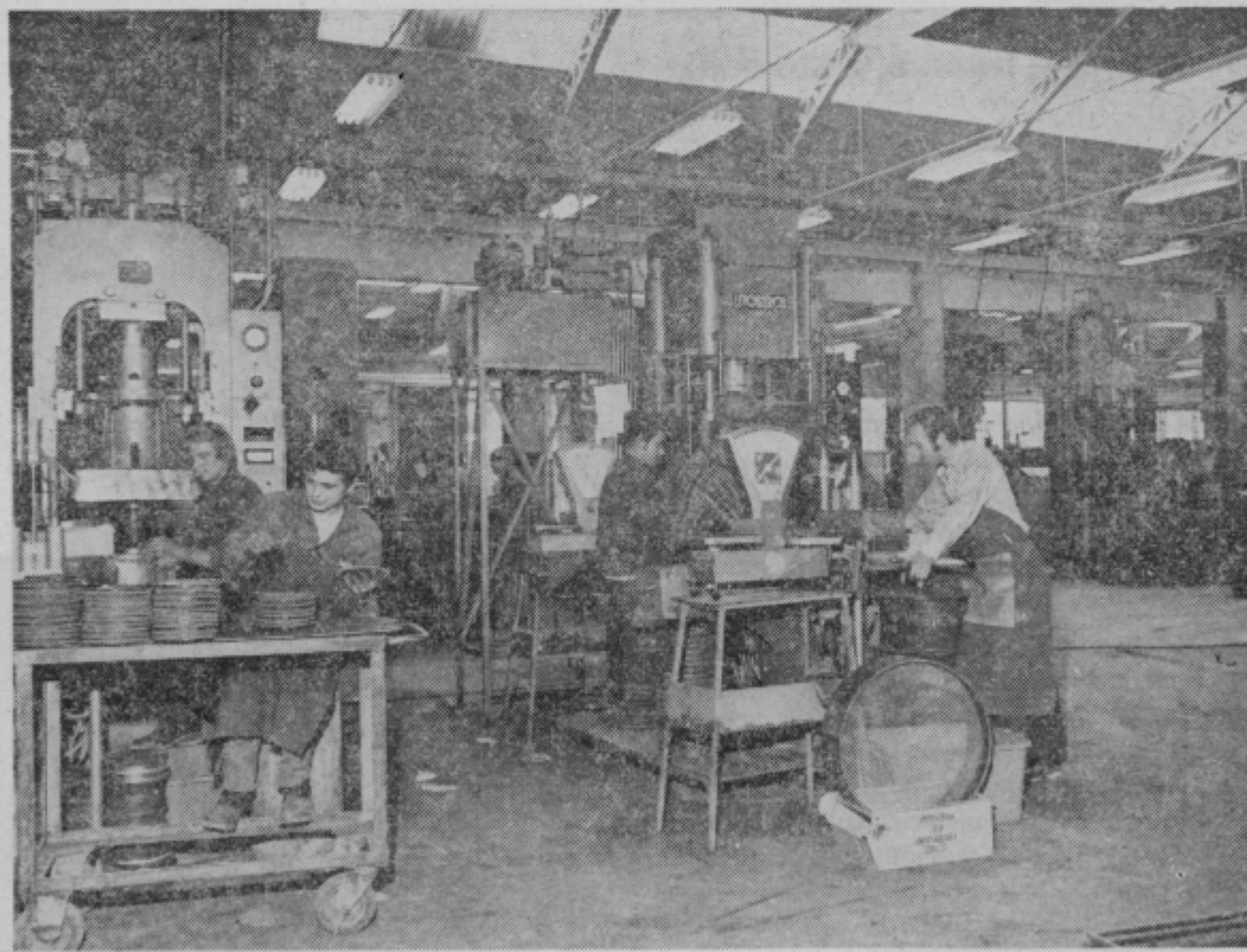
Detajl iz proizvodnje bakelitnih brusov v tozdu Coflex
