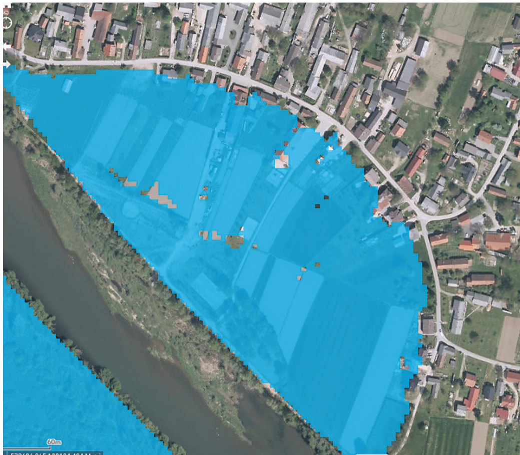
Razlivanje Drave ob stari strugi Drave v Novi vasi pri Markovcih pri pretoku okrog 2.400 m 3 /s. Pri takšni vrednosti pretoka bi bili pod vodo tudi objekti v delu naselja Siget v Stojncih in tamkajšnje farme.
