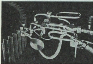
Plamensko kaljenje zobatega kolesa po postopku zob po zob s pomočjo butan-propan ali pa zemeljskega plina
