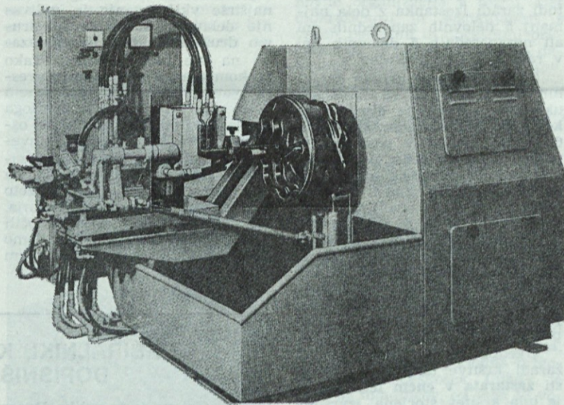
Naprava za indukcijsko kaljenje
