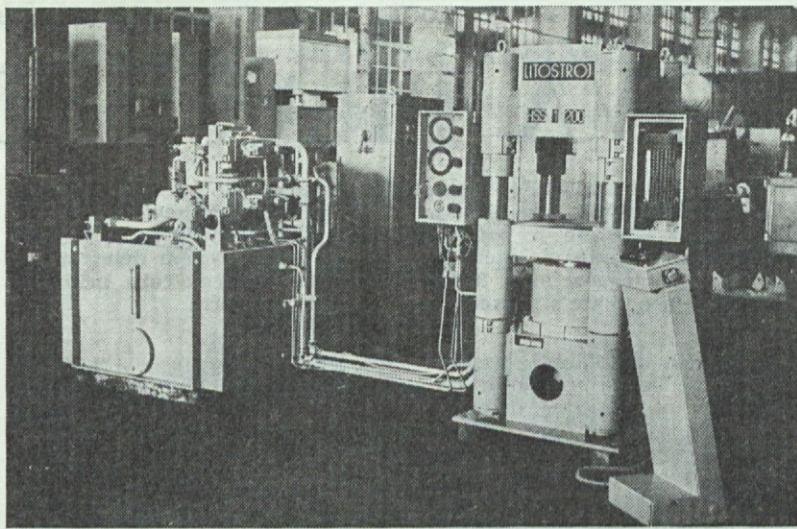
Hidravlični utiskovalnik HSS-1-200... za UNIS-POBEDA Goražde (Foto Zlebnik)
