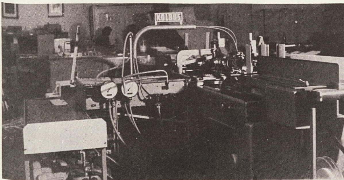
Sodobni avtomatski stroj „Kolbus“ za izdelavo platnic
