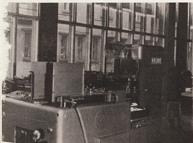
Sodobni avtomatski stroj „Kolbus“ za vplatičenje in dokončno oblikovanje trdo vezanih knjig
