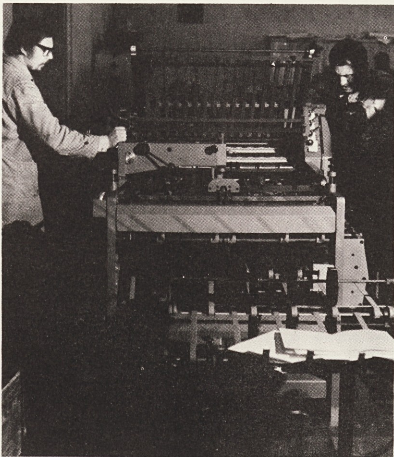
Avtomatski zgibalni stroj tovarne „Stahl“ za zgibanje pol do velikosti 78 x 114 cm za zaporedno in križno zgibanje
