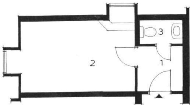
PODSTREŠJE, LOKAL 10: 1. predprostor . . . . . 3,35 m 2 2. delovni prostor . . . 15,50 m 2 3. sanitarije . . . . . 1,85 m 2 Skupaj: . . . . . 20,70 m 2
