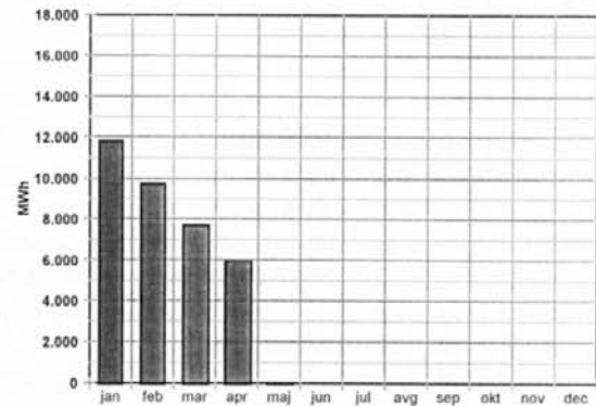
Pregled proizvodnje toplote za centralno ogrevanje za leto 2001
