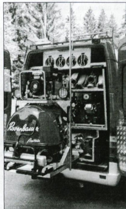
Avtomobil GV-V1 poleg devetih sedežev v potniškem delu vsebuje vse, kar je potrebno za gašenje
