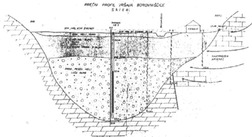
45b. Skica prečnega prereza vodnega zajetja na t. i. Borovniškem vršaju. (S. Jakin).
