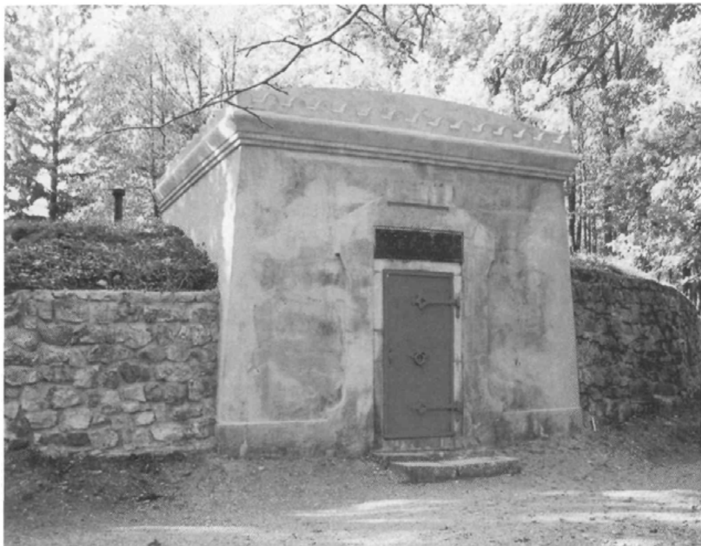
41. Vodohran na Sveti Trojici, zgrajen leta 1904.
