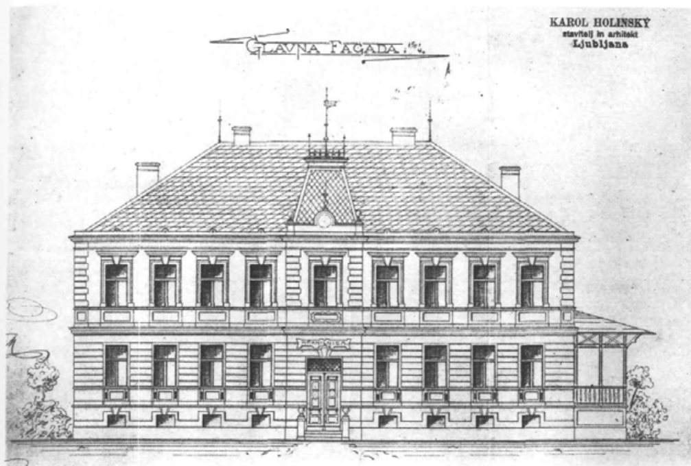
19. Načrt stavbe Kmetске posojilnice, zgrajene v letih 1903–1905.
