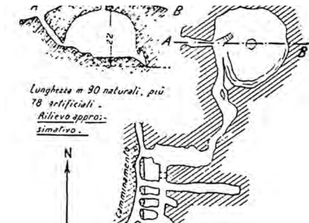
FOTO 29: NAČRT RUSKE JAME. VIR: L. V. BERTARELLI, E. BOEGAN, DUE MILLE GROTTA DI GUERRA , MILANO 1926, 137.
