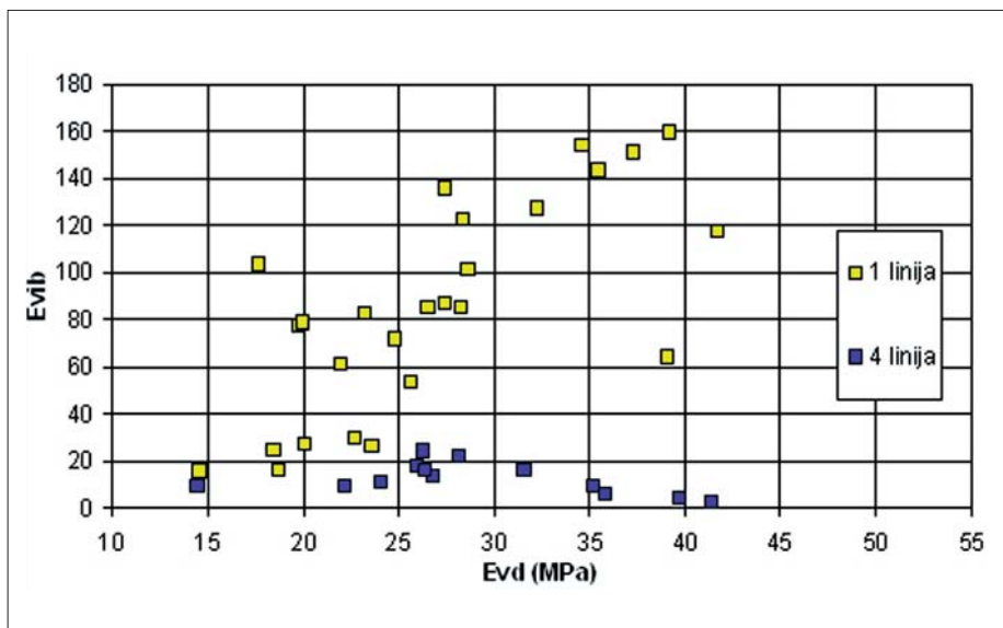
Slika 23 • Rezultati primerjalnih meritev s CCC ( E_{vb} ) in krožno ploščo ( E_{vd} ) pri Dolgi vasi
