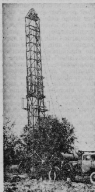
Raziskovalni stolp in aparat na tovarnjaku pri odprtini iz katere bo pritekla topla voda na Turnišču.
