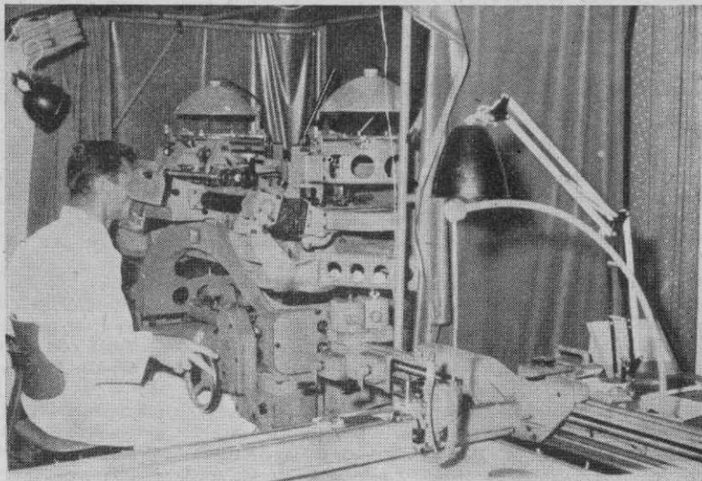
Izdelava načrtov z modernim stereokartirnim aparatom
