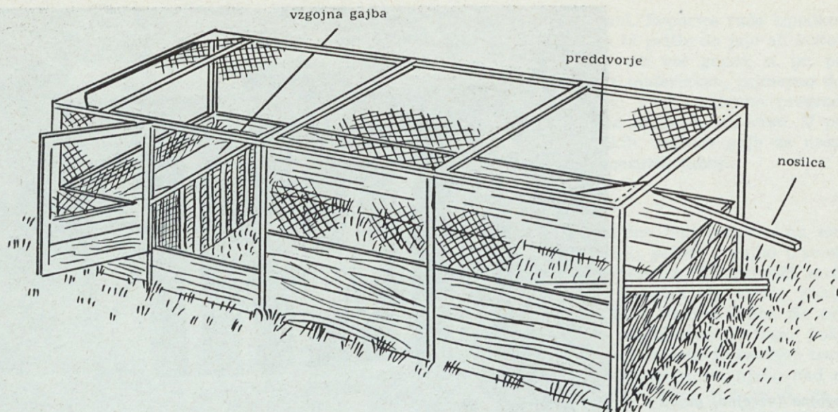
Premakljiva vzrejna (vzgojna) gajba s preddvorjem
