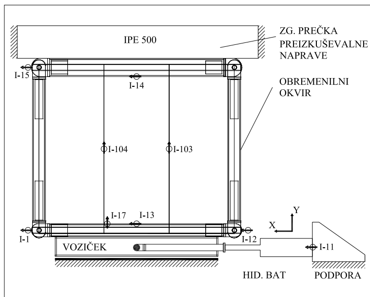
Slika 7 • Postavitev merilcev pomikov
