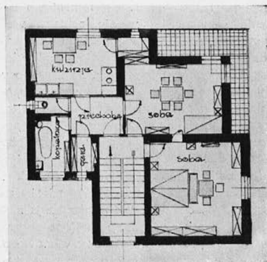
Nadstropje
