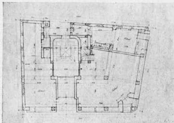
Prizemlje
