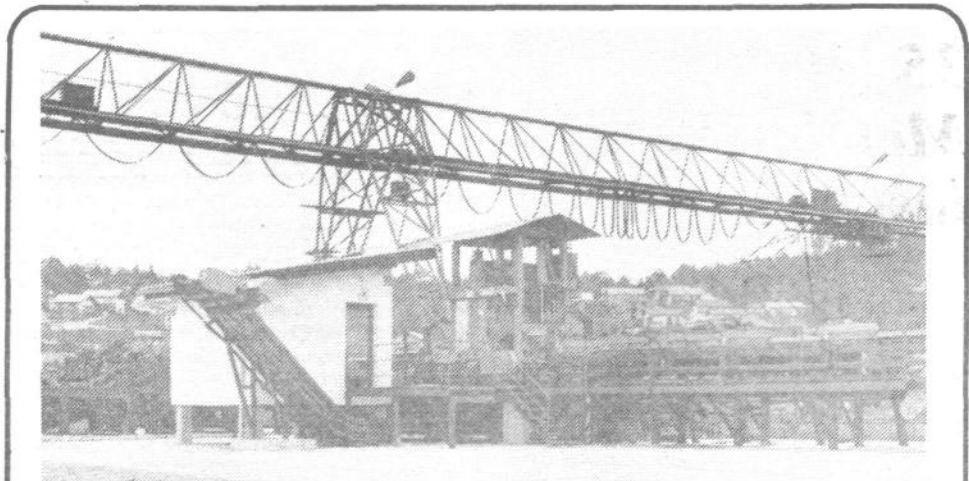
Nova naprava - kakovostno obdelana in razrezana hlodovina - Hojina Žaga na Škofljici je z novo naložbo začela lansko jesen. Linija za razrez lesa je stala 85 milijonov. Ob njej bosta dovolj dva človeka, saj je naprava avtomatska in računalniško vodena.
