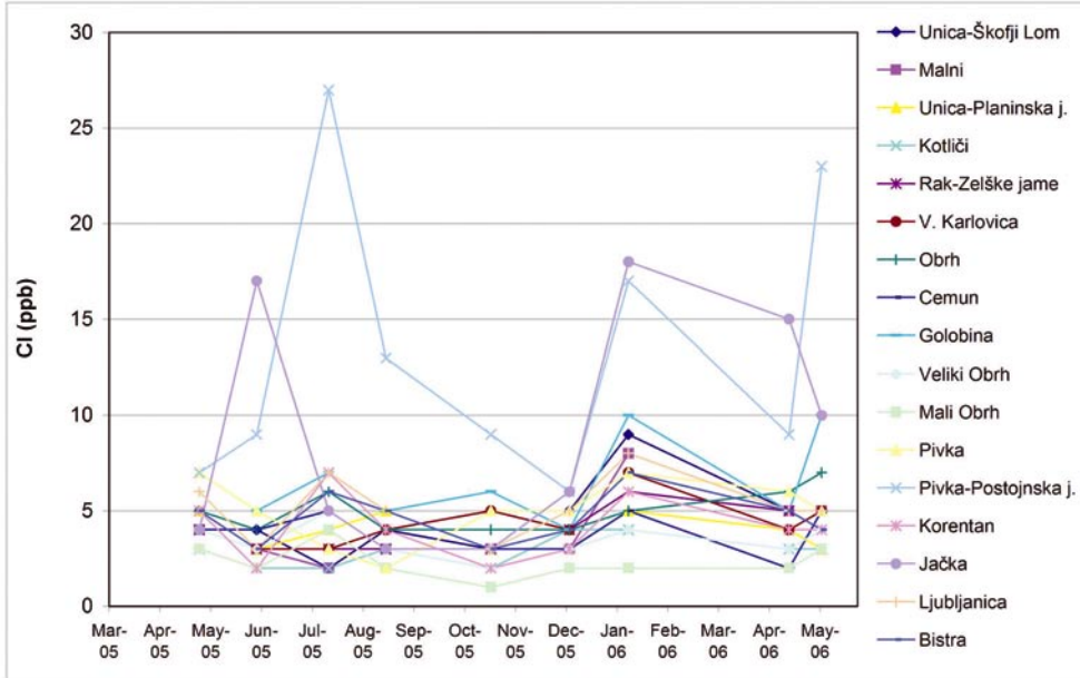
Slika 7. Koncentracije klora v vzorčenih voda v obdobju I. faze monitoringa Figure 7. Chlorine concentrations during the first monitoring phase
