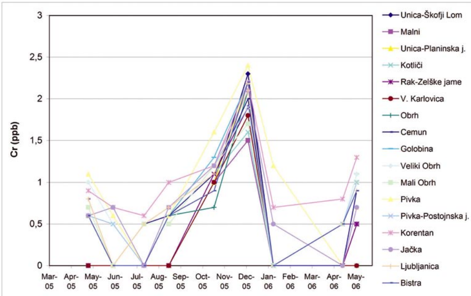
Slika 8. Koncentracije kroma v vzorčenih voda v obdobju I. faze monitoringa Figure 8. Chromium concentrations during the first monitoring phase
