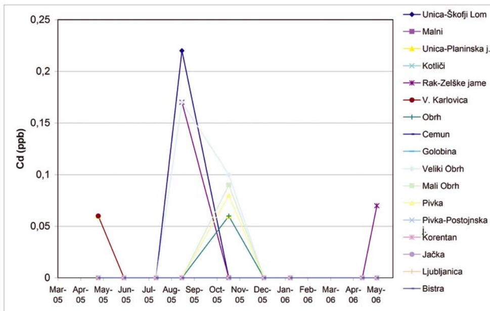
Slika 6. Koncentracije kadmija v vzorčenih vodah v obdobju I. faze monitoringa
