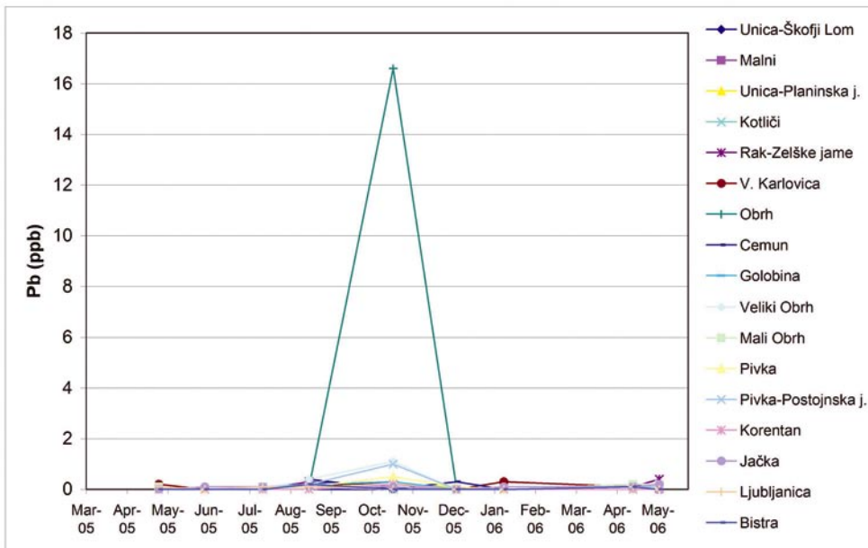
Slika 11. Koncentracije svineca v vzorčenih voda v obdobju I. faze monitoringa
