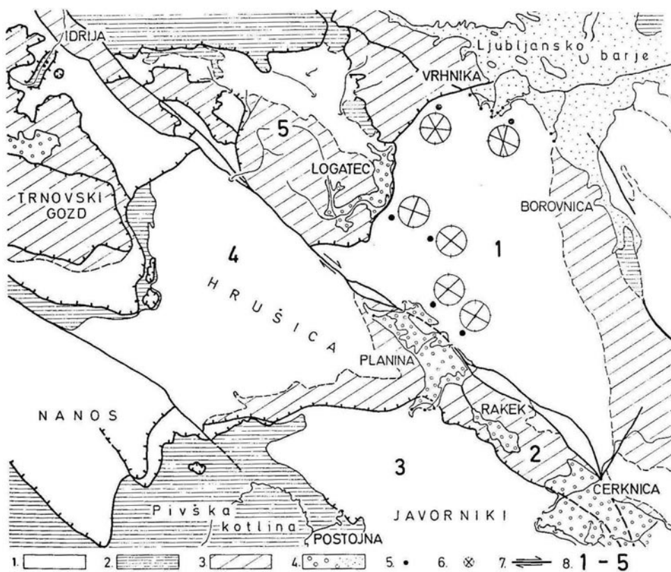
Slika 2. Hidrogeološke enote v srednjem delu kraškega porečja Ljubljane (1 – apnenčev, 2 – neprepustne kamnenine (skrilavci in drugo), 3 – dolomit, 4 – naplavine na kraških poljih in barju, 5 – lokacije merjenih ruptur, 6 – diagrami ruptur, 7 – prelomi, 8 – hidrogeološke enote: (1) Vrhnika-Cerkniška gruda, (2) Rakeško-cerkniška gruda, (3) Javorniško-snežniška gruda, (4) Hrušica, (5) Idrijsko-žirovska pokrovov (Habič et al., 1976)
