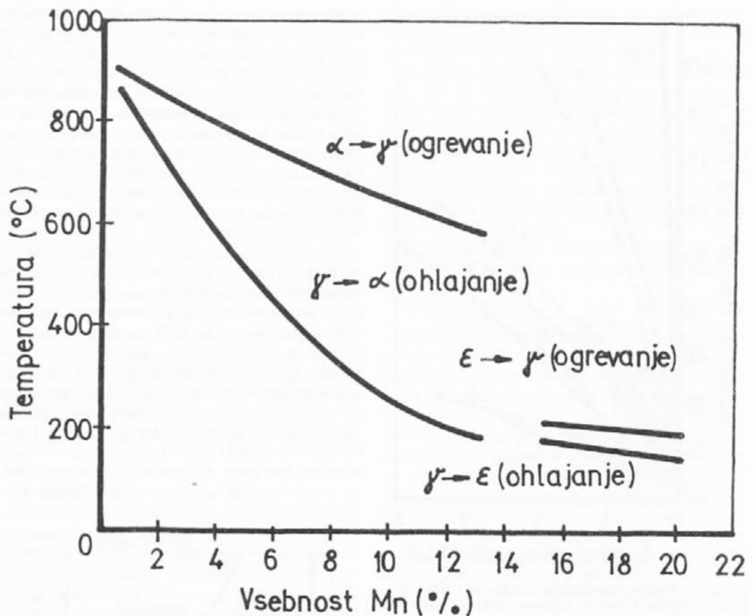
Slika 4: Premeni \delta na faze (oustelita) v \alpha ali \epsilon sta drsni, to je brez sprememb vsebnosti mangana. Strukturi sta nestabilni, spominjata na martenzit v drugih jeklih. \epsilon faza je ob tem še neferomagnetna.
