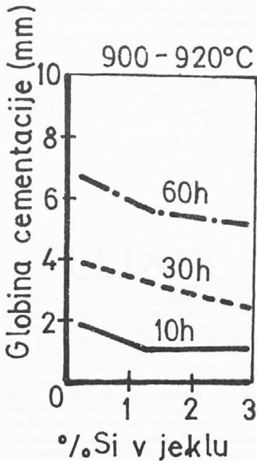
Slika 2. Zmanjševanje globine, do katere množično prodrejo ogljikovi atomi med nagljičenjem pri 900-920°C v času do 60 ur
