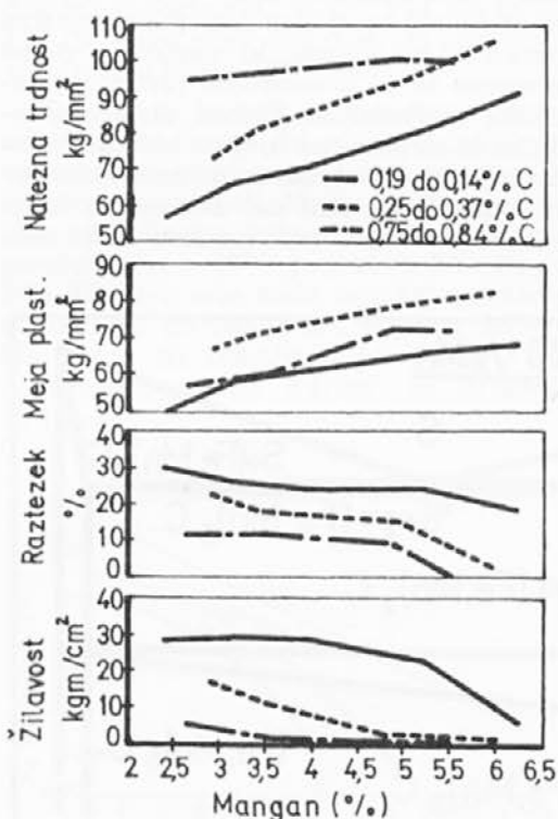
Slika 2: Vpliv povečanja vsebnosti mangana v treh različnih jeklih v 0,09 do 0,84% C na trdnost in plastičnost teh jekel. Več C in Mn normalno povečuje trdnost in napetost, pri kateri se začne stalne deformacije ter zmanjšuje možnost raztegovanja ali upiranja udarcem. Izjema je npr. jeklo z 0,25 od 0,37% C, ki je elastično do najvišje napetosti, celo do 800 N/mm 2 .
