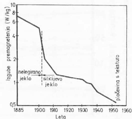
Slika 9. Izgube zadelj premagnetiziranja transformatorske pločevine. Vidno izboljšanje jekla vsaj do 1960. leta
