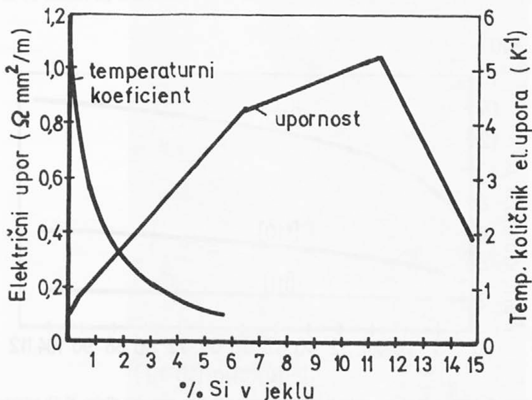
Slika 6. Vpliv silicija na specifično električno upornost jekla in temperaturno odvisnost te upornosti
