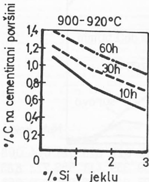
Slika 4. Zmožnost površine izdelka za sprejemanje ogljika med cementacijo pri 900-920°C
