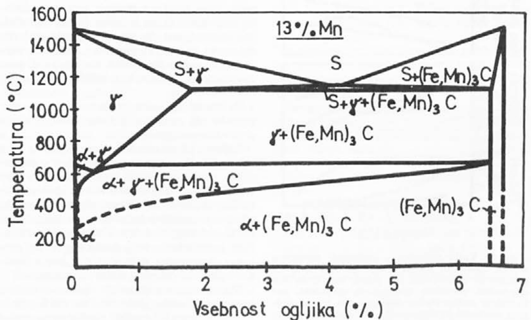
Slika 5: Takoimenovani diagram stanja jekla so 13% mangana. Vidimo precejšnjo podobnost z diagramom Se — C — ni pa za peritepske reakcije.
