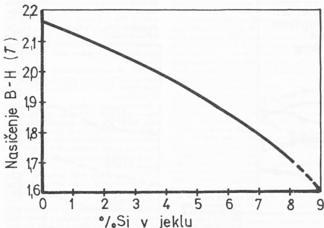
Slika 7. Silicij zmanjšuje možno magnetno nasičenje. Tudi močno magnetno polje ne more namagnetiti silicijevega jekla
