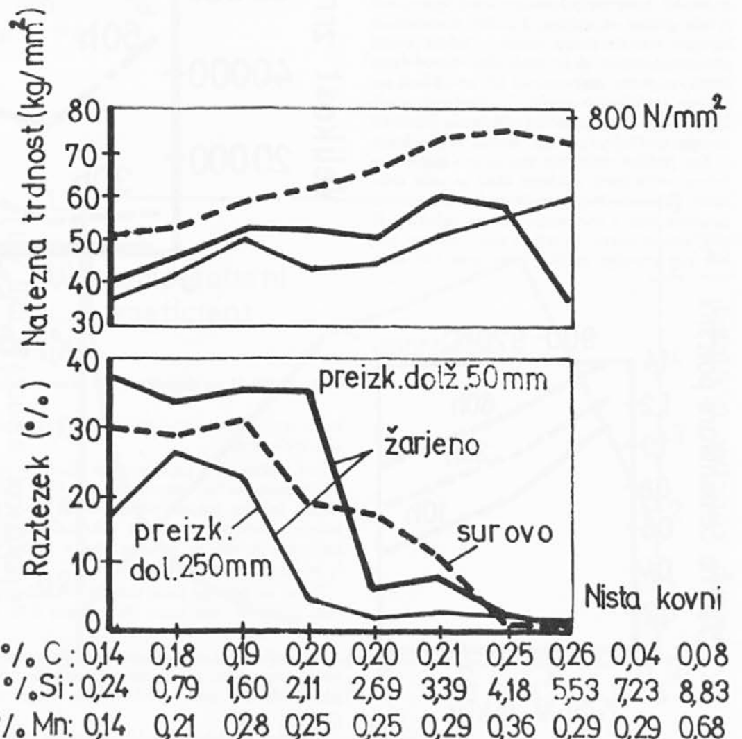
Slika 1. Silicij povečuje trdnost, predvsem pa silno poslabša zmožnost jekla, bodisi surovega bodisi žarjenega, za raztegovanje. Če je več kot 3% Si, pade ta zmožnost na desetino
