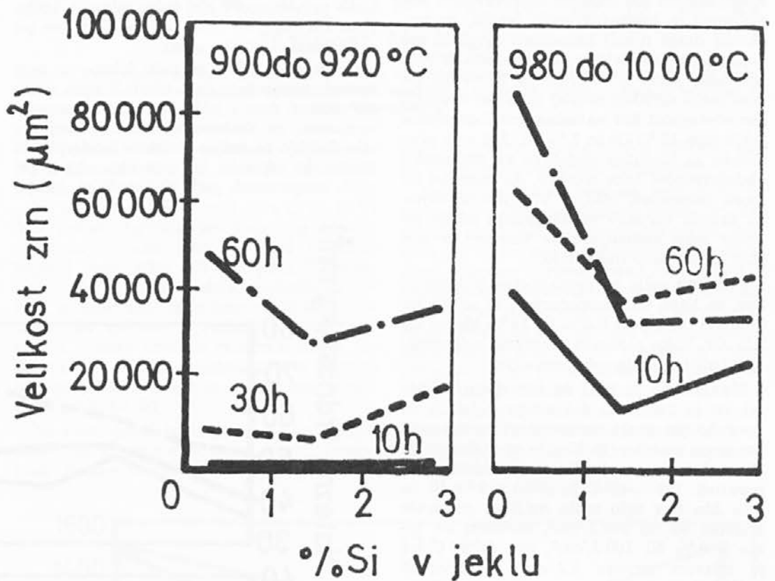
Slika 3. Silicij ne dopušča rasti zrn, četudi jeklo zelo dolgo grejemo pri visoki temperaturi
