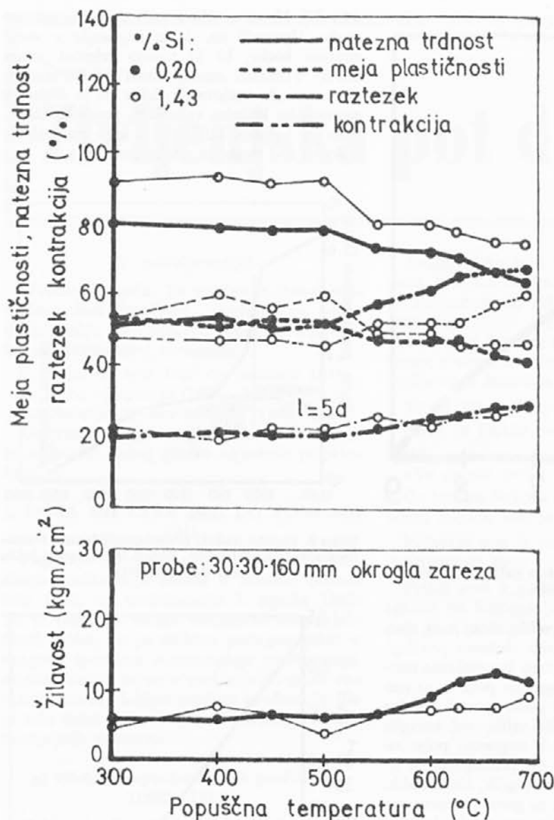
Slika 5. Popuščene krivulje nelegiranega in s silicijem legiranega jekla. Silicij zboljša vse lastnosti razen kontrakcije (zmožnosti za stanjšanje med nateznim preizkusom) in žilavosti po visokem popuščenju
