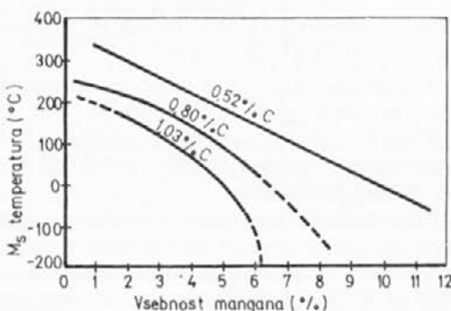
Slika 6: Mangan in ogljik znižujeta temperaturo, pri kateri se med kaljenjem ustvari martenzit (temperatura M s ). Če se tvori še v hudem mrazu, npr. pri -100°C, mu pomagamo priti tako, da jeklo pač hladimo v zadosti mrzlem sredstvu, lahko pa dobimo martenzit tudi s hladno deformacijo (točenjem), čeprav se pri kaljenju še ni prikazal.
