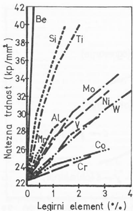
Slika 1: Kako povečujejo različno veliki dodatki različnih kovin natezno trdnost čistemu železu (feritu). Silicij je na drugem, mangan pa na četrtem mestu, za dragima perilijem in titanom ter za silicijem. Molibden in aluminij tekmujeta z manganom.
