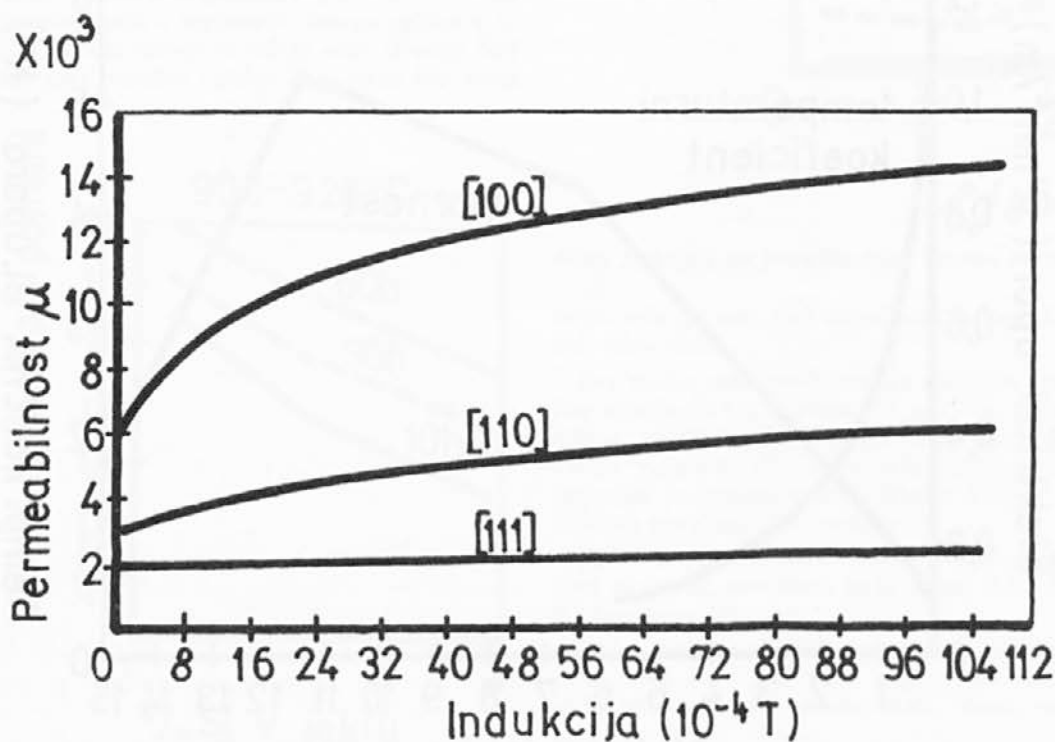
Slika 8. Permeabilnost monokristala zlitine železa s 4% Si za magnetne silnice, ki jih ustvarjamo z indukcijo. Smer (100) pomeni vzporednost k robu kocke osnovne celice, (110) ploskovno diagonalo, (111) prostorsko diagonalo osnovnih celic v jeklenem zrnju
