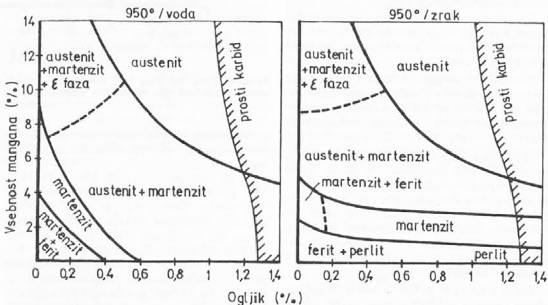
Slika 3: Strukture manganovih jekel: Perlitna ali avstenitna ali martenzitna ali bajinitna (ni vrisana). Uporabni sta skoraj samo perlitna ali avstenitna, ter martenzitna teh jekel ni lahko popustiti, da bi ga mogli mehansko obdelati. Vidimo, da je že malo mangana zadosti, da tudi kaljenje na zraku oblikuje čisti martenzit.
