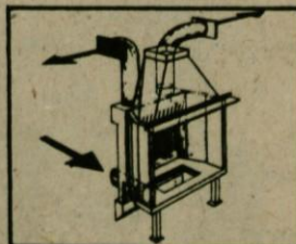
elementi odprtega kamina s sekundarnim ogrevanjem zraka
