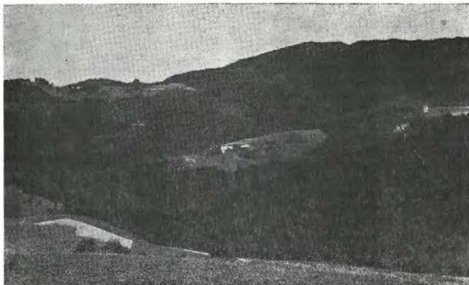
Sl. 43. Pogled iz vasi Vinharje proti močno razčlenjenemu svetu v povirju Hotoveljske. V terasi nad Drnovškovo kmetijo, na sredini slike gledamo najstarejše ostanke pleistocenskega površja. Po tej dobi je prevladala erozija, ki je izdelala skupaj z denudacijo tudi široke zatrepe v povirjih posameznih grap
