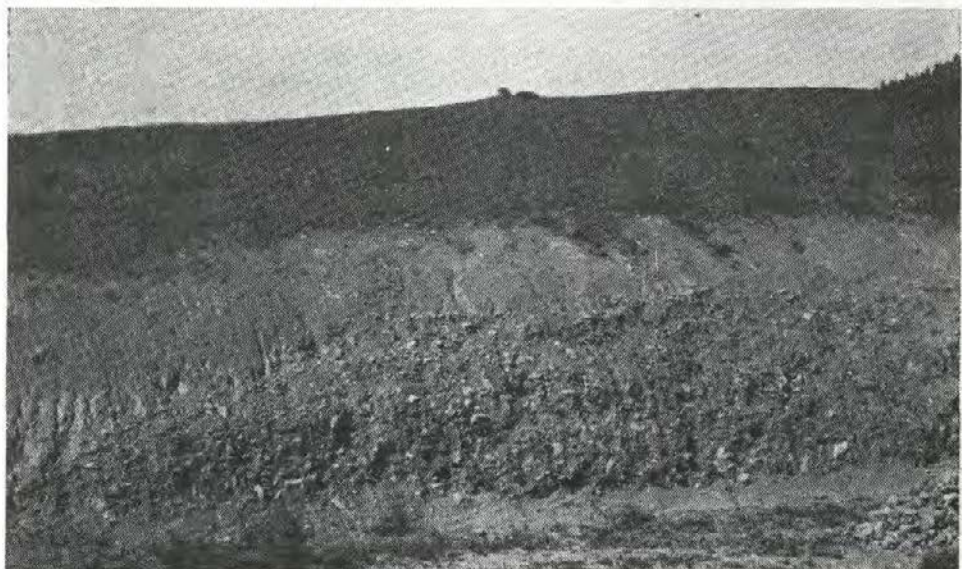
Sl. 38. Tako debel prod je nasul v vasi Selo potok Zabrežnik izpod Žirovskega vrha v mindelski ledeni dobi (terasa 3)
