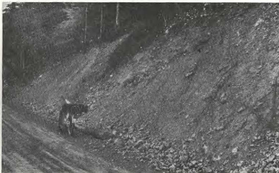
Sl. 10. Tako debele plasti opniškega periglacialnega drobirja je razkrila nova cesta nad Selškimi Lajšami, ki pelje iz Kroke proti Dražgošam
