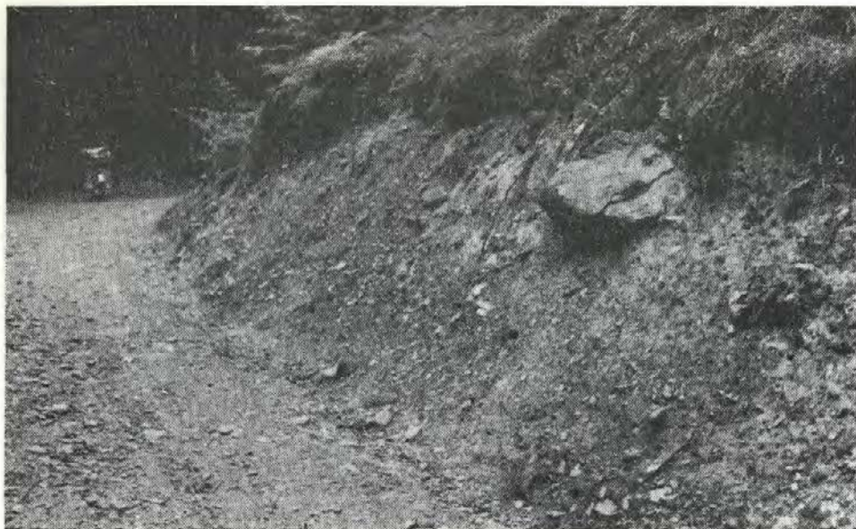
Sl. 45. Tako debel in slabo zaobljen prod pokriva teraso 4 nad Gabrkom
