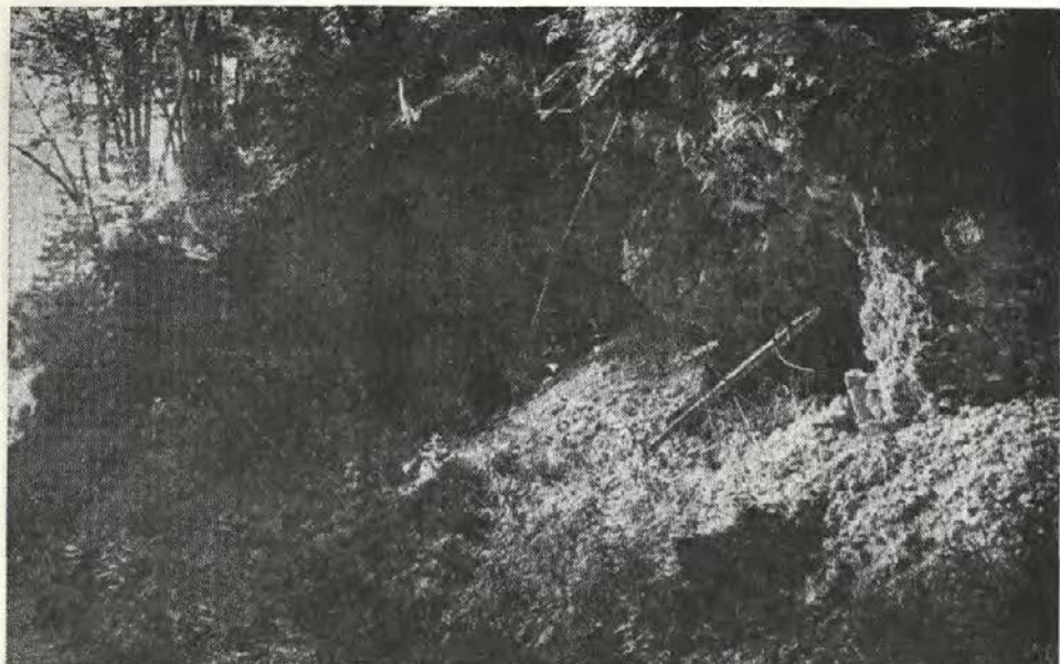
Sl. 27. Tako v brečo zlepljen drobir je razkrit ob poti, ki pelje po pobočjih Jelovice iz Dražgoš proti zahodu
