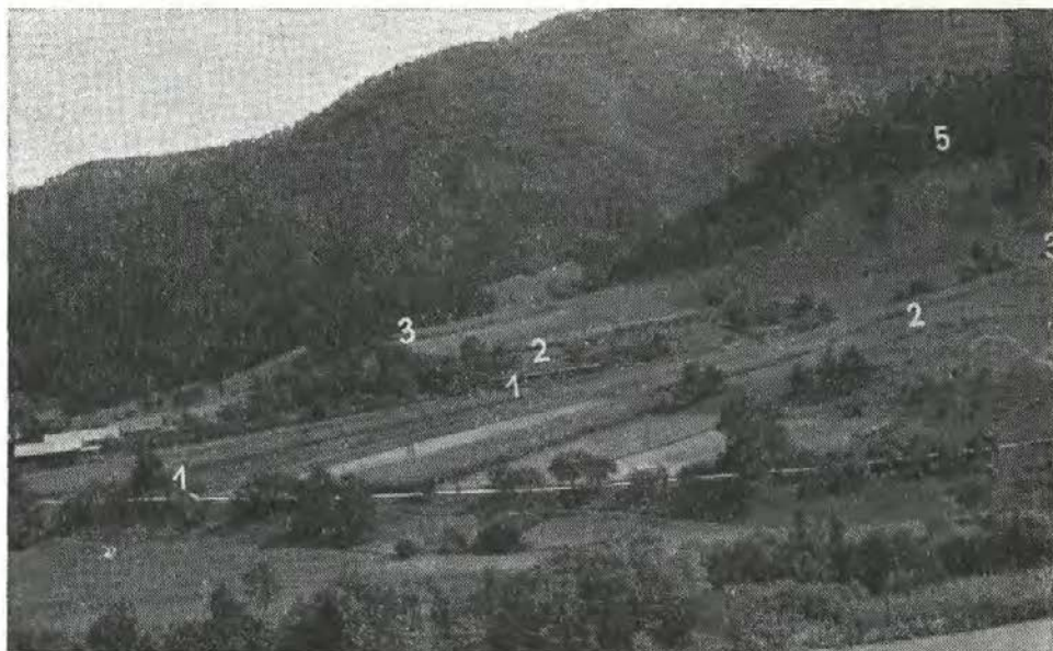
Sl. 22. Pogled čez Poljansko dolino proti Logu. Na sredini slike je velik vršaj, ki ga je v zadnji ledeni dobi nasul potok izpod Valterskega vrha (terasa 1). Nad njim sledijo ohranjeni deli vršajev oziroma teras iz starejših poledenitvenih obdobj (2, 3 in 5)
