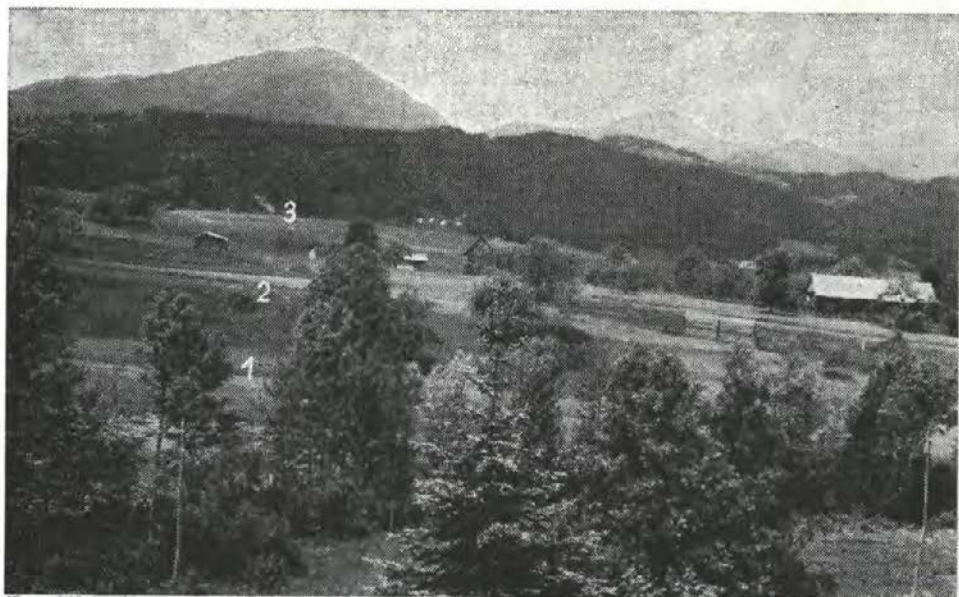
Sl. 31. Pogled po razrezanih ledenodobnih vršajih potoka Dršaka v Gorenji Dobravi (terase 1, 2 in 3)
