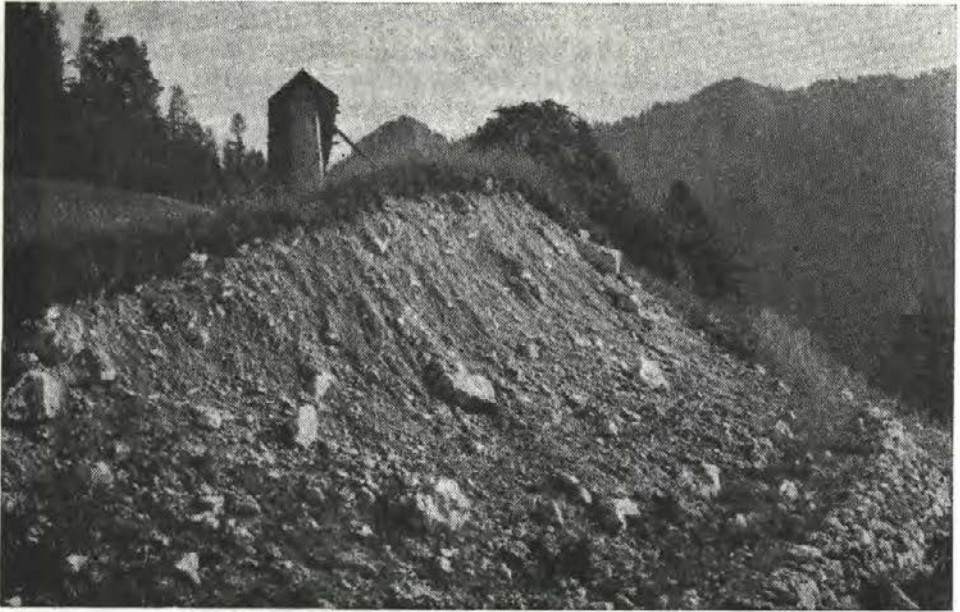
Sl. 2. Cesta, ki pelje iz Sorice proti Podbrdu, se globoko zareže v würmski morenski nasip in nam na široko razkriva njegovo sestavo
