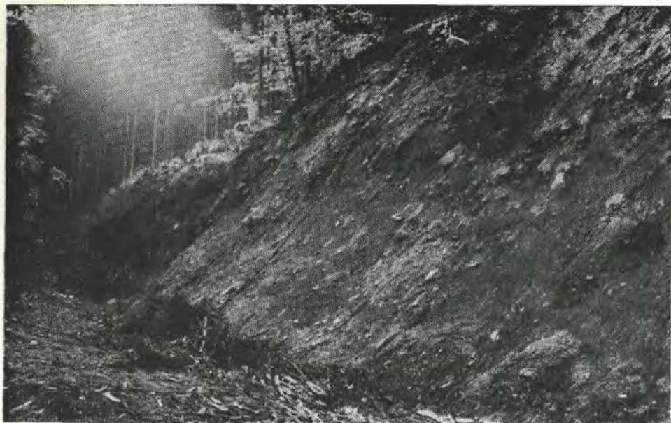
Sl. 4. Tako debele plasti soliflukcijskega gradiva so razkrili pri gradnji nove ceste po dolini Dašnice
