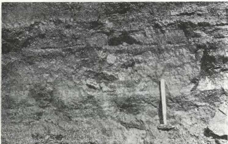
Sl. 24. Značilna drobna plastovitost peščenih ilovic in peskov v Gregorčičevem opekarniškem koku v Virmašah pri Škofji Loki
