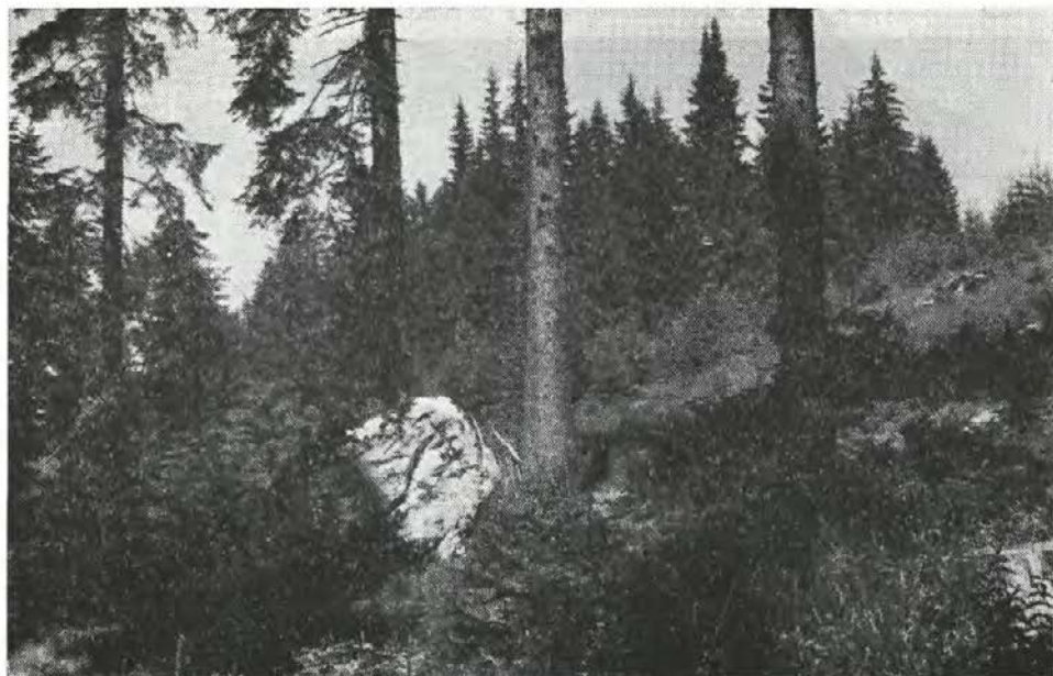
Sl. 6. Pogled na enega od balvanov na morenah bohinjkega ledenika pod Jesenovcem (1218 m), južno od Ledin na Jelovici
