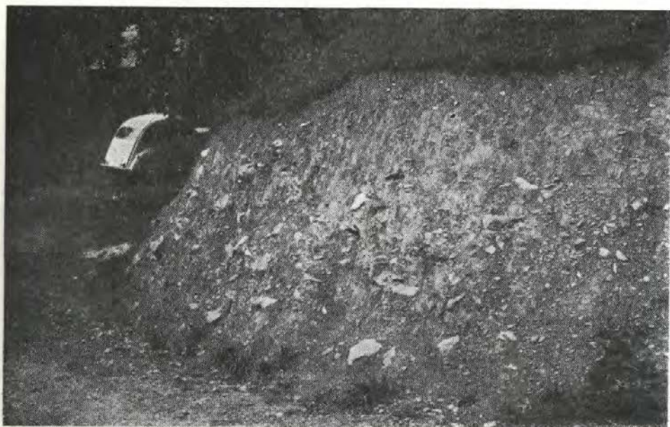
Sl. 18. Tako slabo zaobljen prod sestavlja vršaje v vasi Podpreval v dolini Ločivnice
