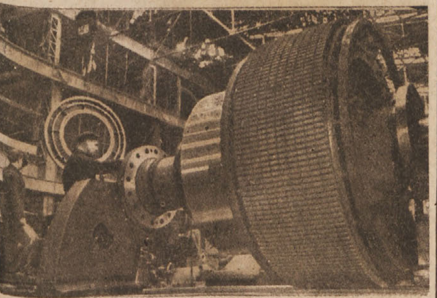
Gradnja največjega turbogeneratorja na svetu v leningrajski tovarni »Elektrosila«
