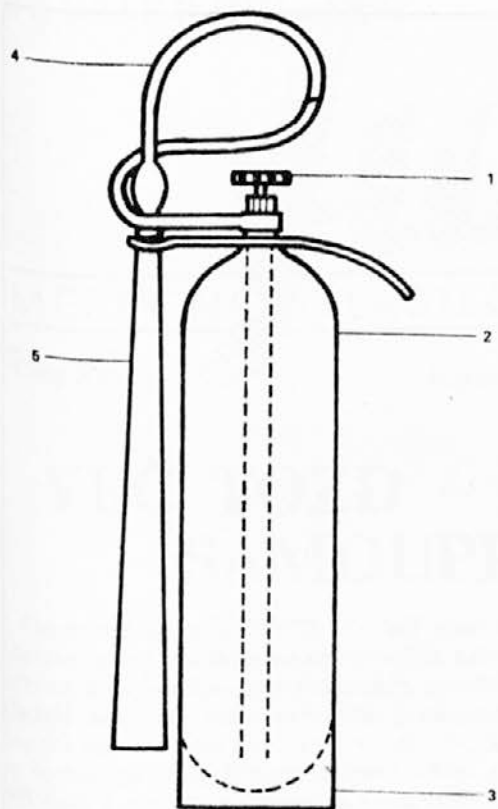
Skica 2 — 1 kolo za odpiranje jeklenke, 2 jeklena posoda, 3 ojačeni del spodnjega dela jeklenke, 4 gumijasta armirana cev, 5 ročnik
